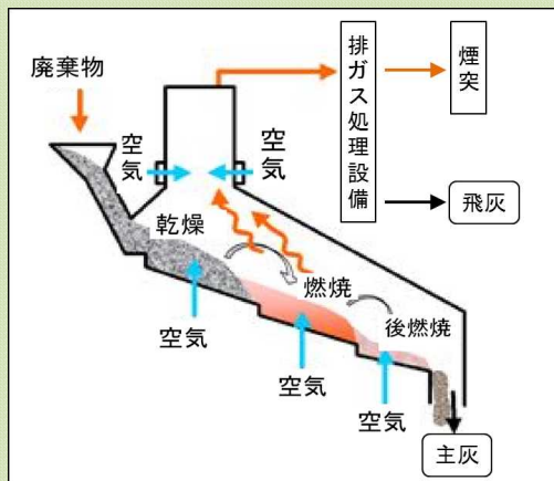
ストーカ式焼却炉の概略
